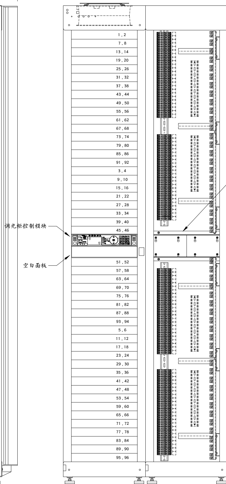
2 正视图
