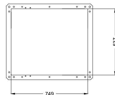
3 仰视图
