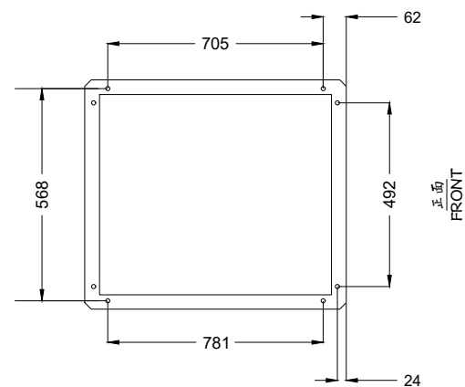
4 地板安装位置
