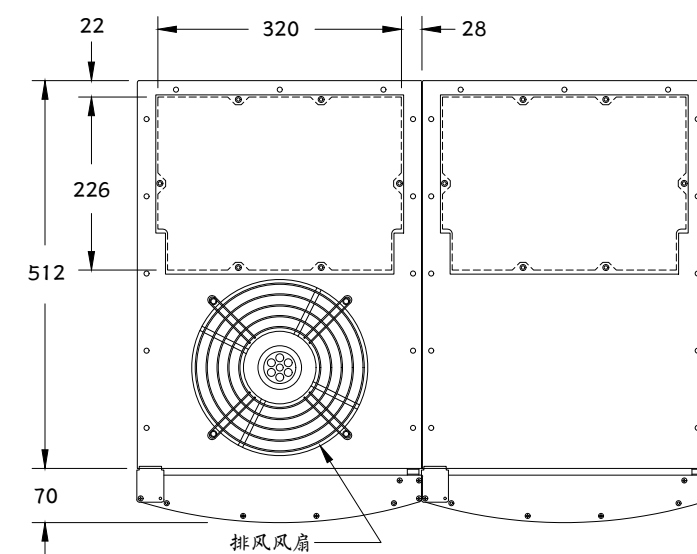
4 仰视图
