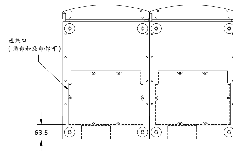
5 俯视图
