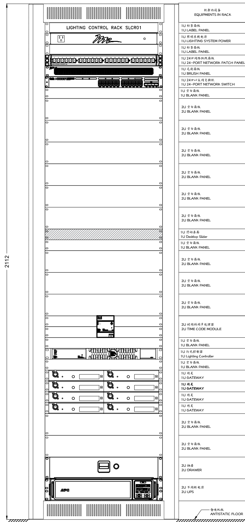
1 正视图
