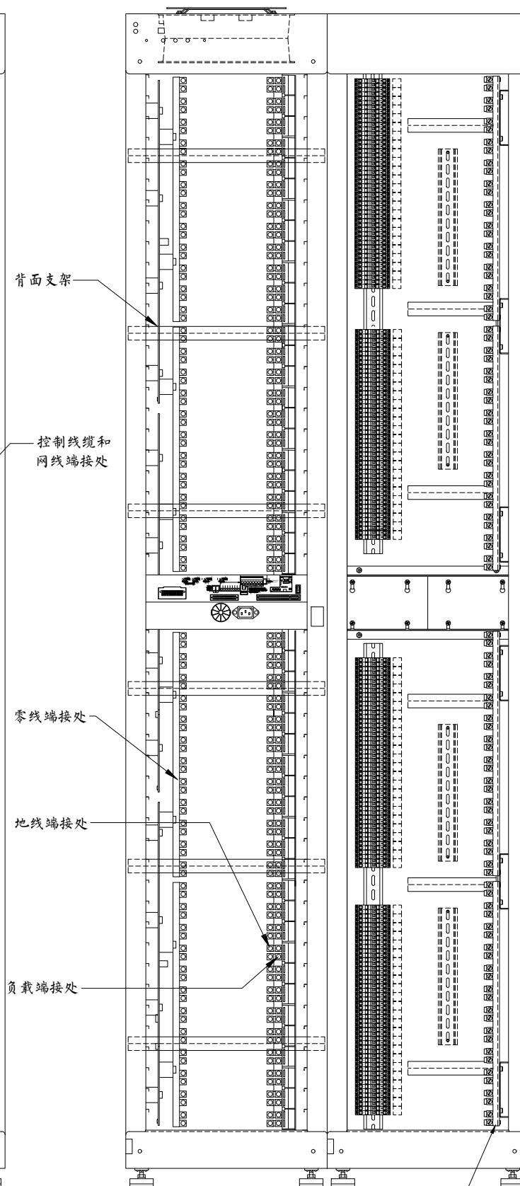
3 正视图(模块移除)
